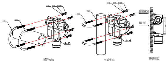
图 4-1 安装示意图
