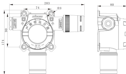
图 2-1 外形尺寸示意图（单位：mm）
