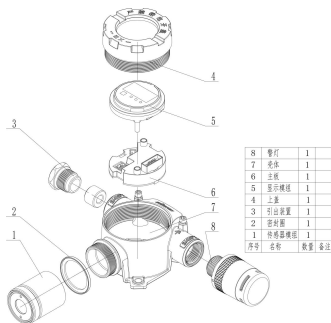
图 2-2 组成结构示意图
