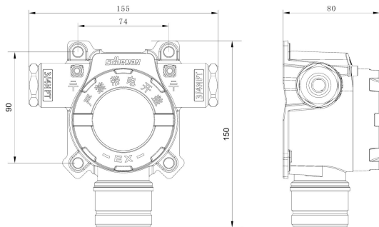
图 2-2 SST610 系列外形尺寸示意图（单位：mm）
