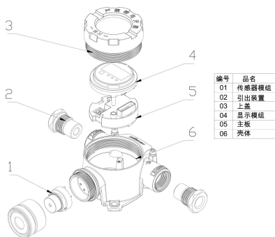
图 2-6 SST610 系列组成结构示意图
