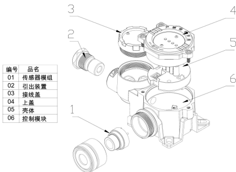
图 2-5 SST607LED 系列组成结构示意图
