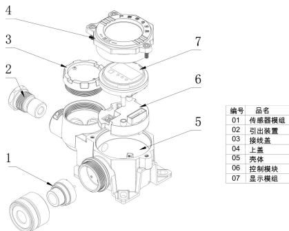
图 2-4 SST607LCD 系列组成结构示意图
